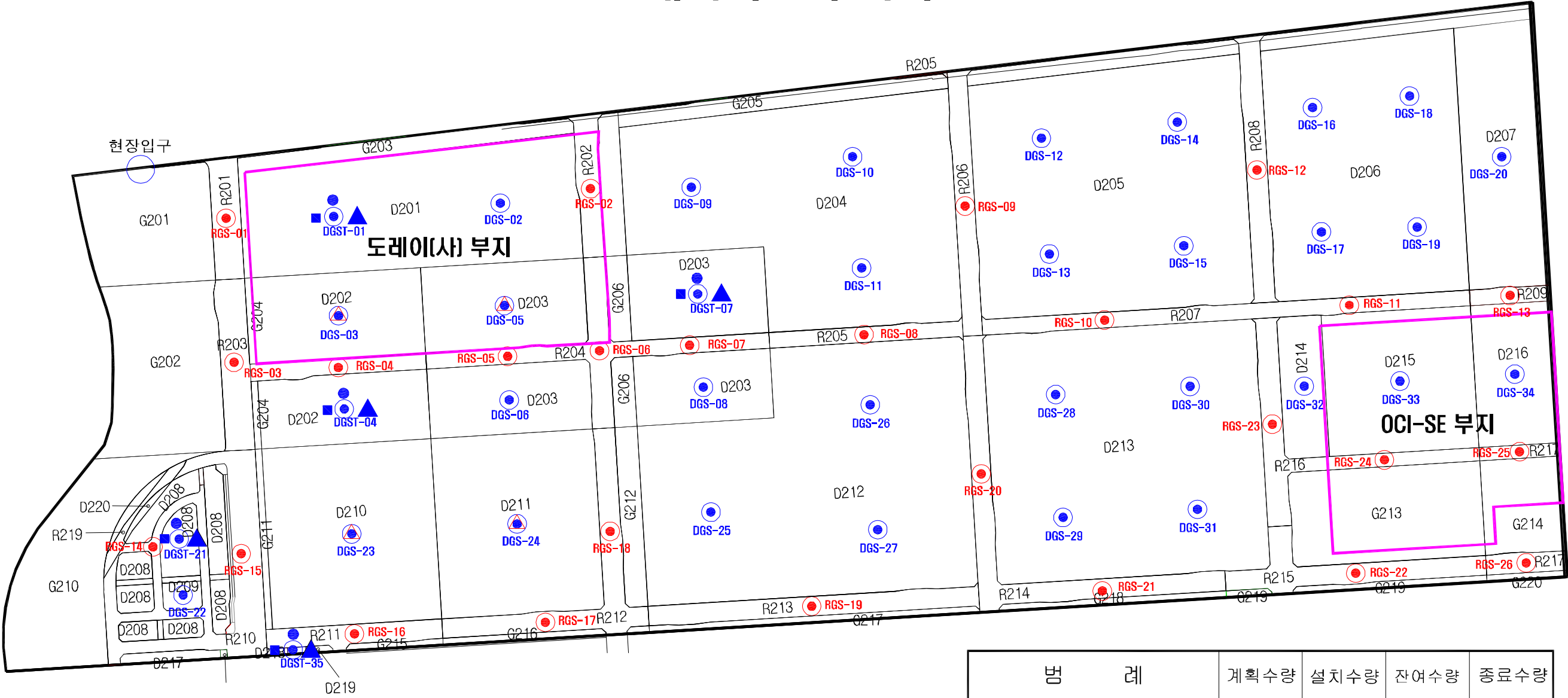
계측기설치 위치도
